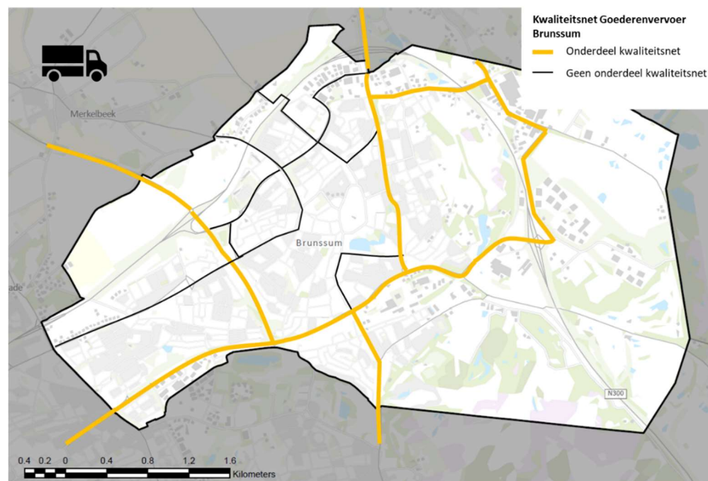
Figuur 10. Kwaliteitsnet Goederenvervoer Brunssum
